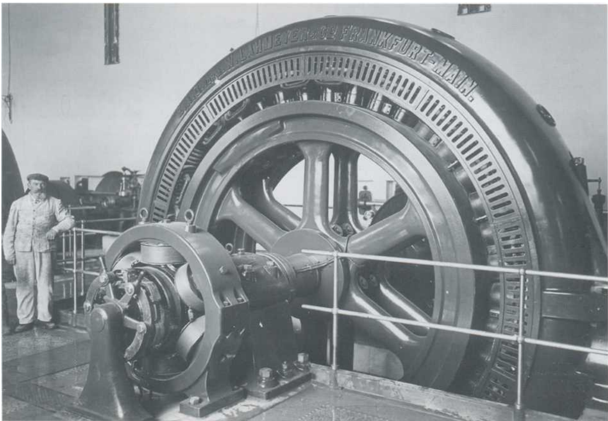
Maschinenhaus, Generator 1 '500 PS 21. April 1904
