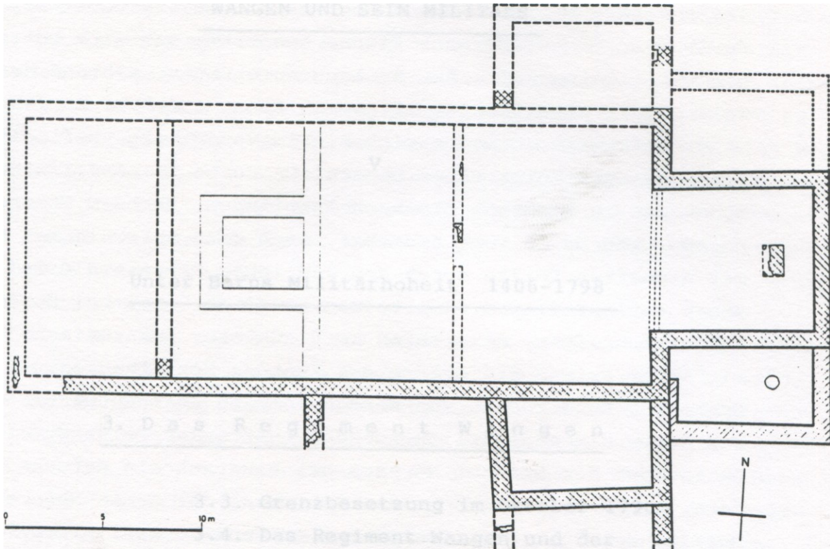
Grundriss der Anlage II. M. 1:250.
